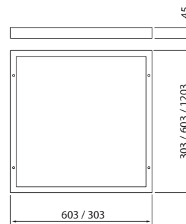
Pinta-asennuskehyset
