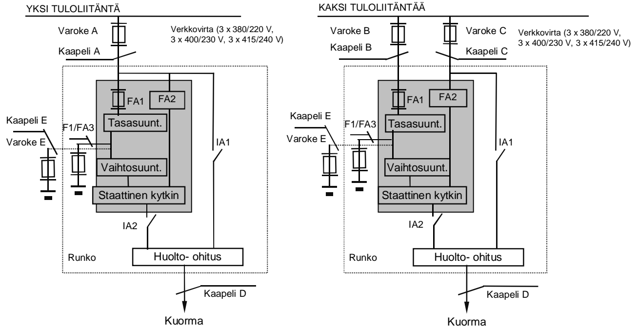
Kuva 3. Lohkokaavio, POWERSCALE 10–50 kVA
