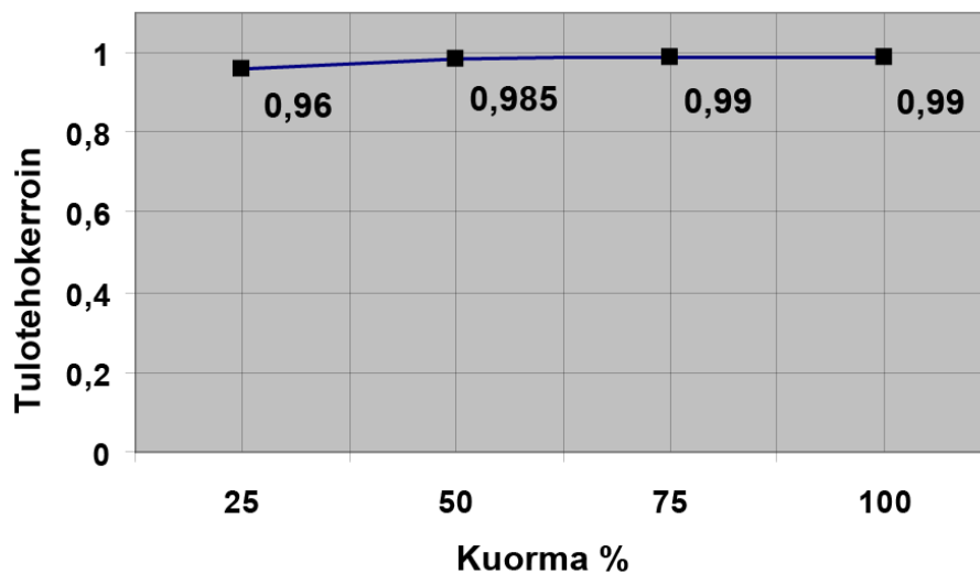
Tulotehokerroin (kapasitiivinen)
