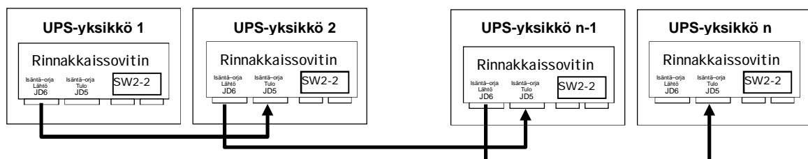
Kuva 1.2. UPS-yksiköiden rinnankytkentä: väyläkaapeliin kytkeminen rinnakkaissovittimien välille.
