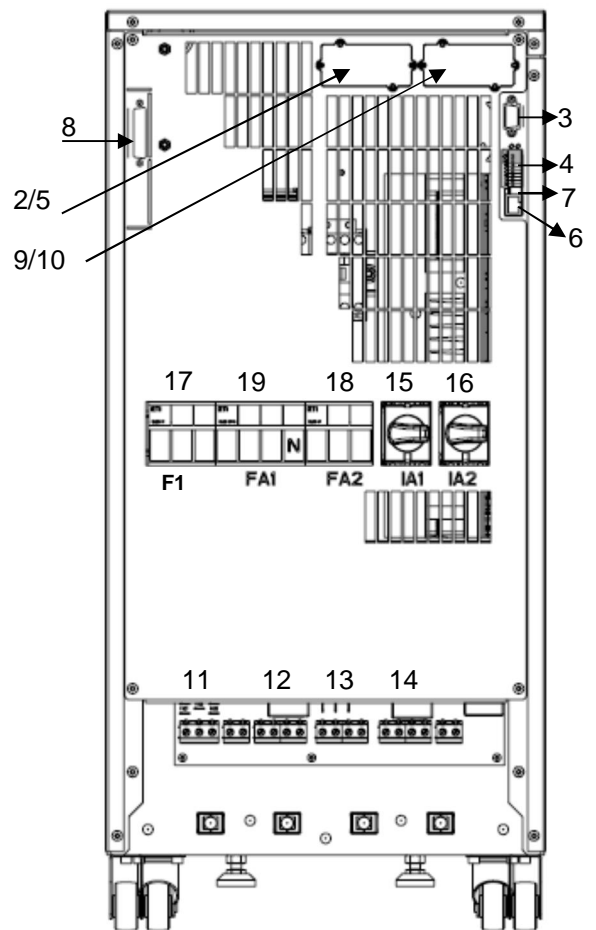
NÄKYMÄ TAKAA
