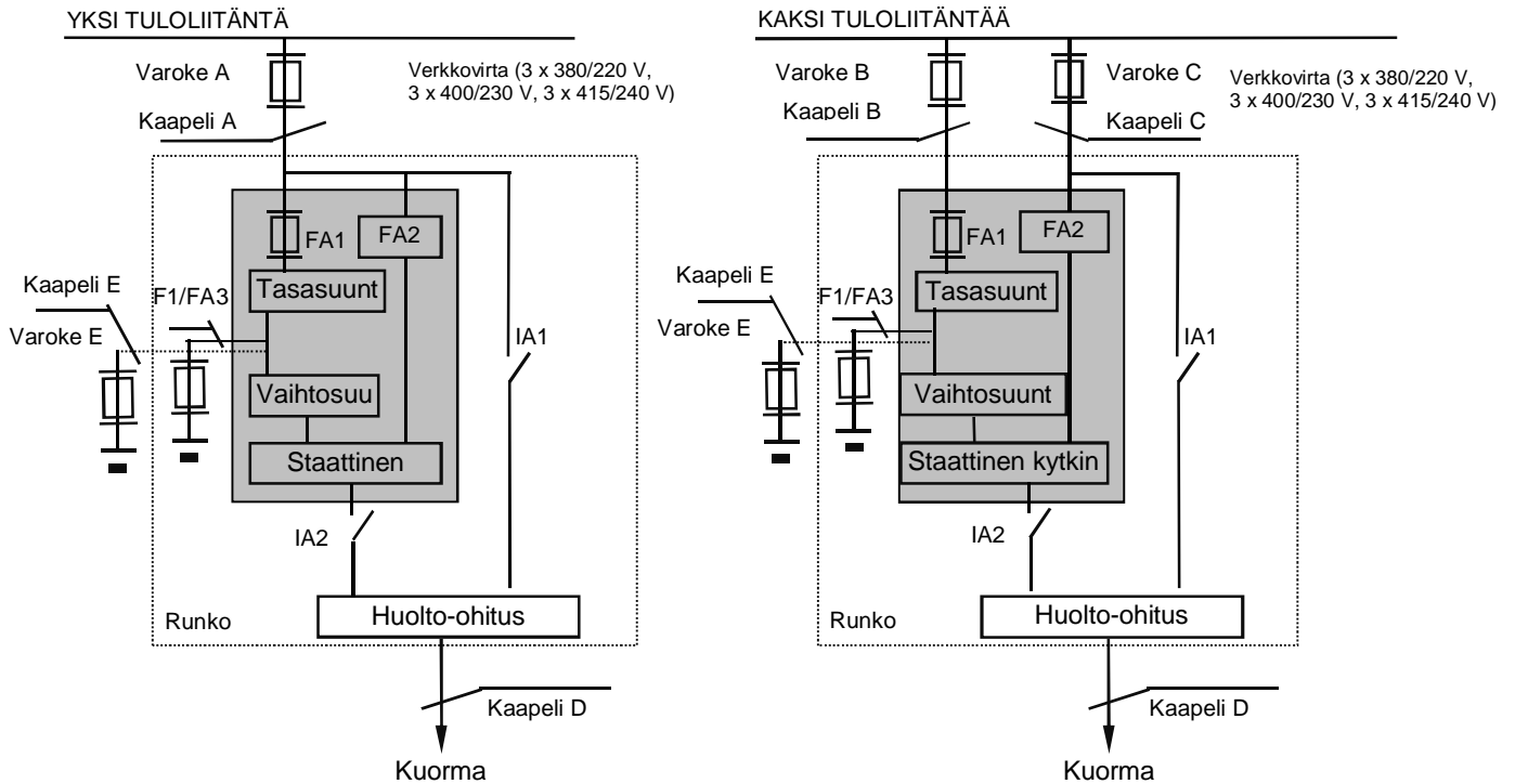
Kuva 3. Lohkokokaavio, POWERSCALE 10–50 kVA
