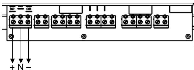
Kuva 4. Ulkoisten erillisten akustojen kytkeminen.
