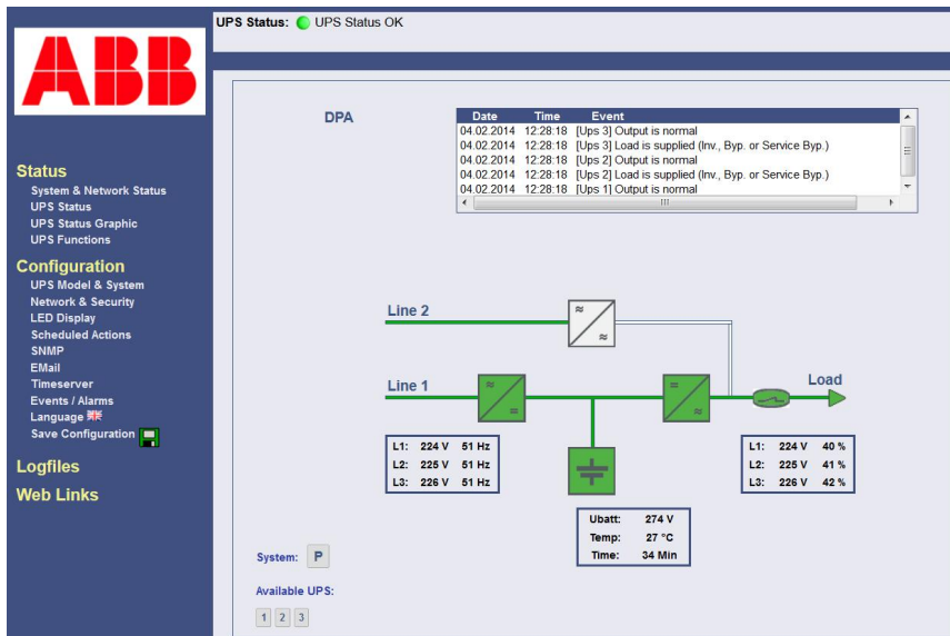
Kuva 1.4.2. Valvontanäkymä.
