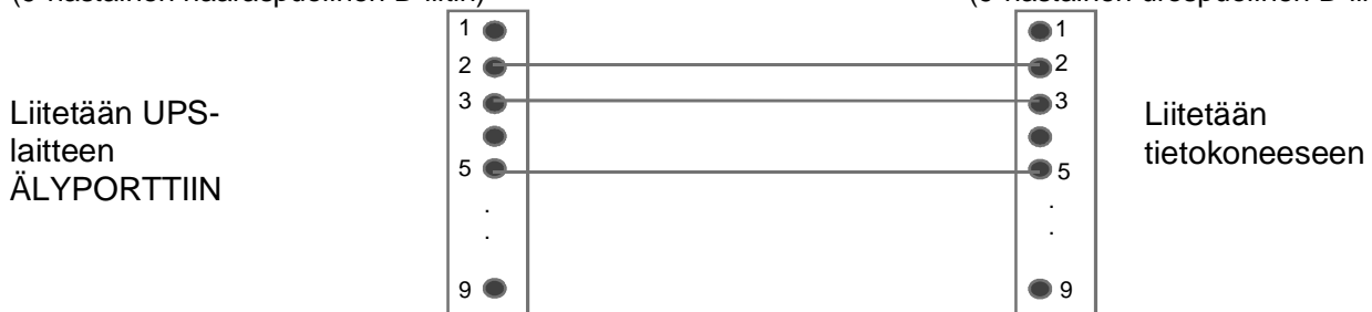
Kuva 1. Liitäntäkaapeli – 9-nastainen sarjaporttiliitin
